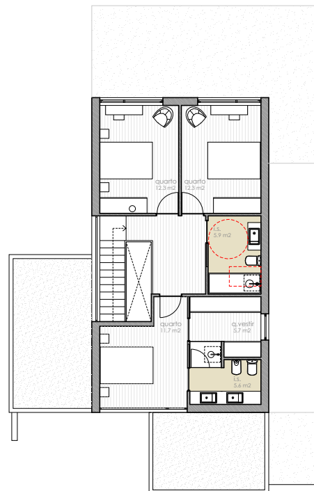
PLANTA PISO 1
