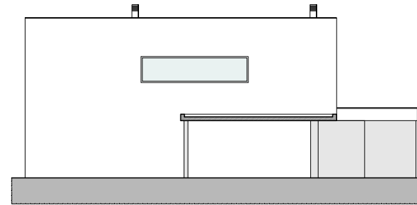
ALÇADO LATERAL 1
